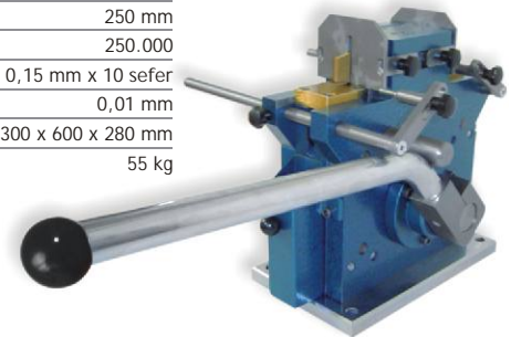
UN-03 KÖPRÜLEME Önlü - Arkalı köprüleme makinesi
