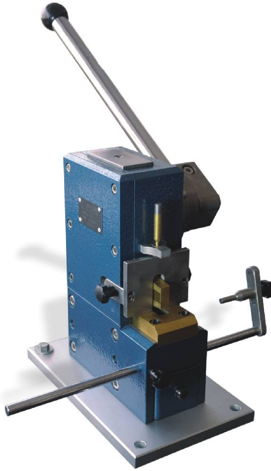
UN-04 KÖPRÜLEME Köprüleme makinesi
